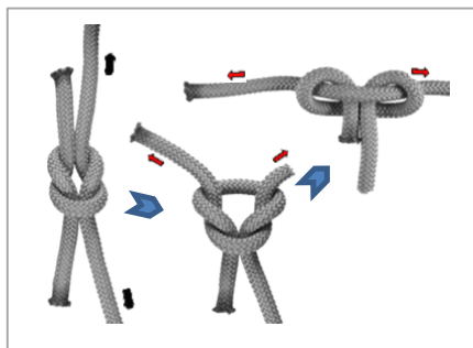
Figuur 10. Het kantelen van een vaste platte knoop naar een schuivende leeuwerikskop. De zwarte pijlen geven een normale last aan waarbij de knoop intact blijft. Wanneer aan de uiteinden wordt getrokken (rode pijlen) kan de knoop kantelen en eindigen als een schuivende knoop, zoals een leeuwerikskop.
