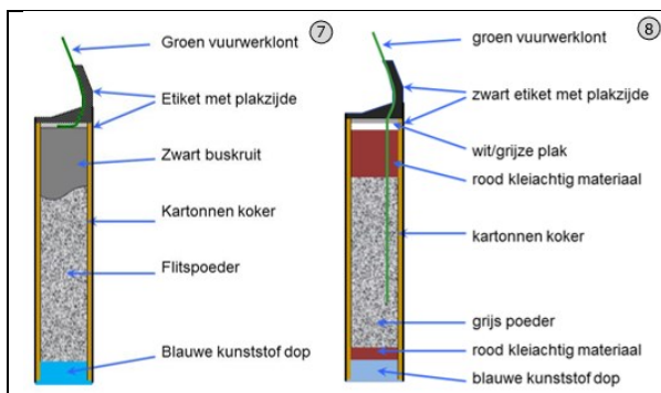
Figuur 7. Schematische opbouw van de Super Cobra 6 van foto 1. Figuur 8. Schematische opbouw van de Super Cobra 6 van foto 5.
