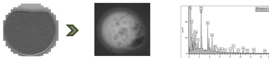
Figuur 3 - De automatische SEM/EDX analyse bestaat uit twee fasen. (1) de deeltjes op een oppervlak (stub) worden in kaart gebracht. (2) van kandidaat schotrestdeeltjes wordt per deeltje de elementsamenstelling bepaald aan de hand van het röntgenspectrum. Na de automatische analyse worden ook de vorm en afmetingen (steekproefsgewijs) onderzocht.
